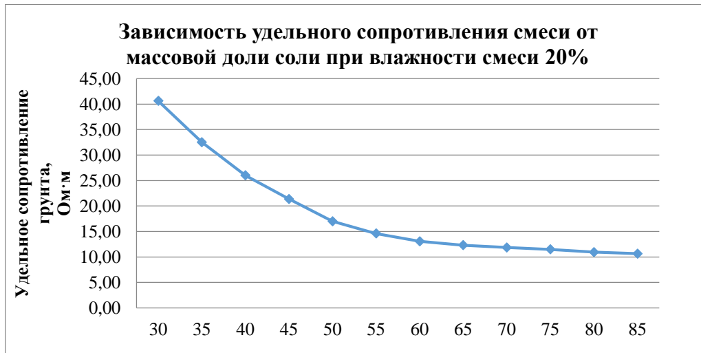
Рисунок 5. Зависимость удельного сопротивления смеси от массовой доли соли.
