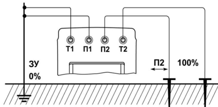
Рисунок 2. Схема измерения сопротивления заземления экспериментальных электродов при помощи ИС-10.
