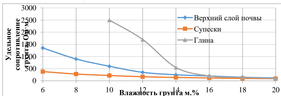
Рисунок 4. Зависимость удельного сопротивления смеси от влажности.
